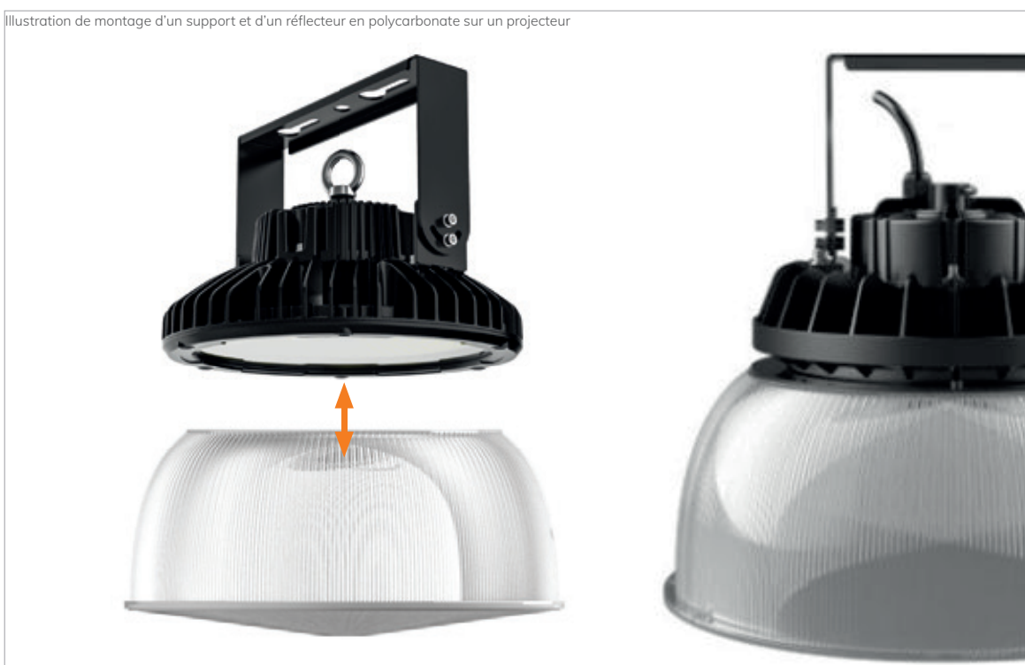
Illustration de montage d'un support et d'un réflecteur en polycarbonate sur un projecteur
