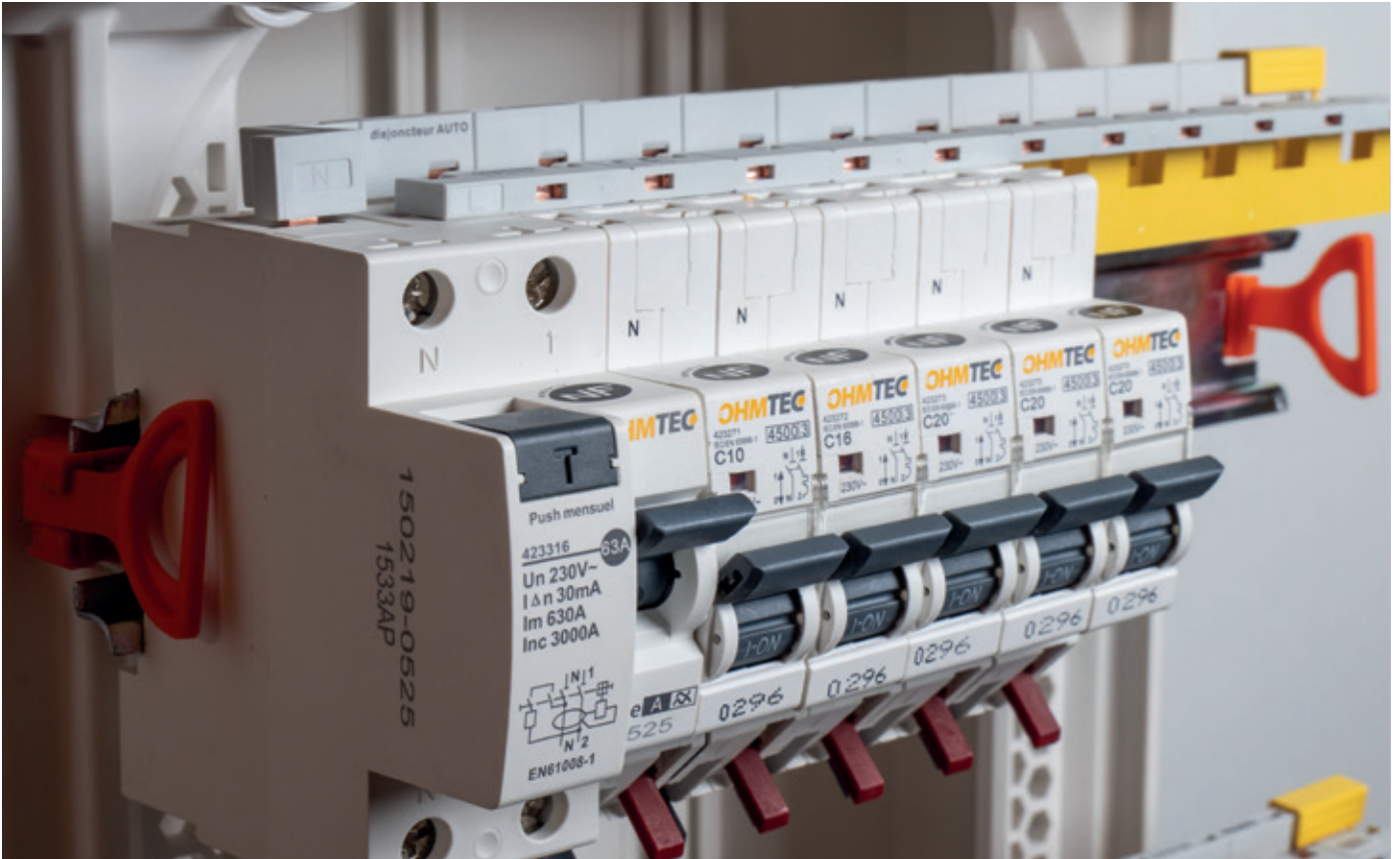
Illustration de montage de la barre de pontage universelle L et N sur disjoncteurs automatiques
